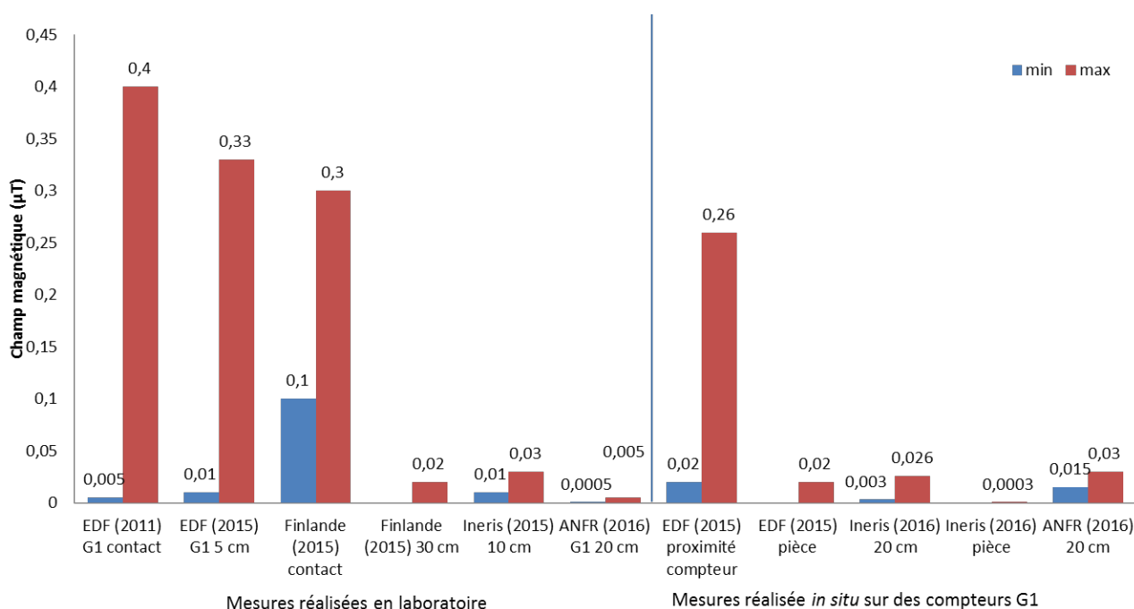
Figure 26 : valeurs de champ magnétique obtenues lors des différentes campagnes de mesures
